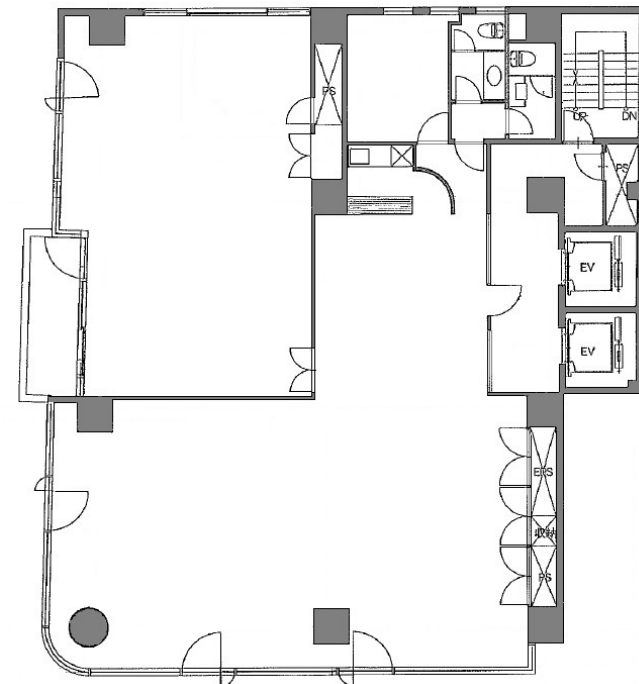
【平面図】
