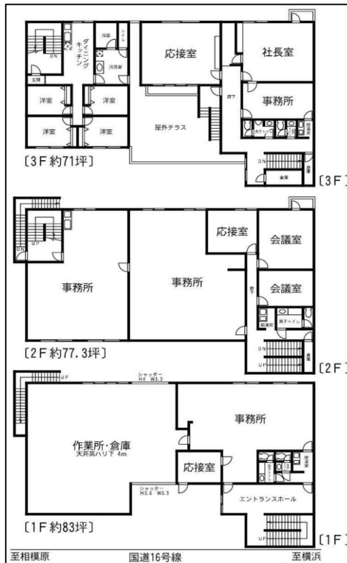
間取図
