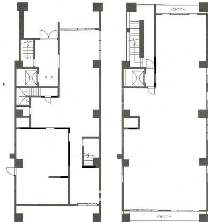
【6F平面図】
